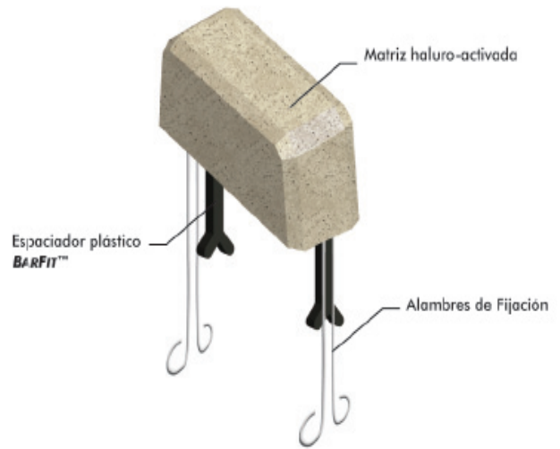
Corte transversal Ánodo Galvanode VP
