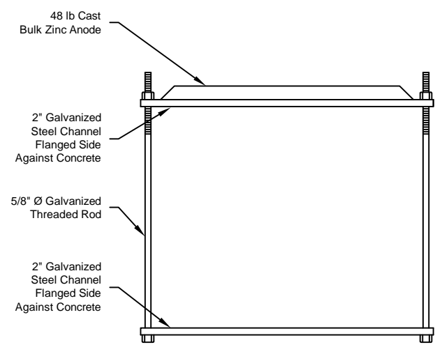
BULK ANODE ASSEMBLY N.T.S.
