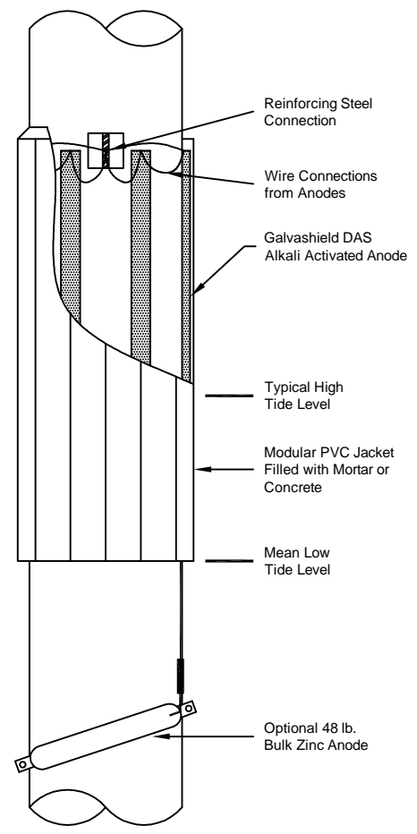
GALVASHIELD DAS JACKET ELEVATION N.T.S.
